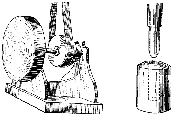
Шлифовально-полировальный круг
