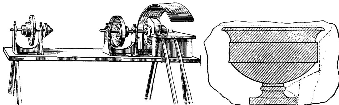
Токарный станок для вытачивания крупных изделий.
